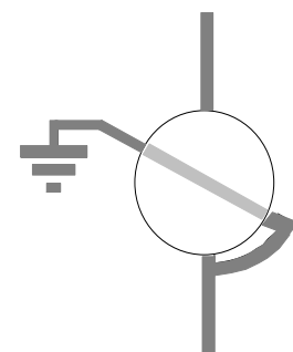
Odpínač vypnutý Uzemňovač zapnutý
